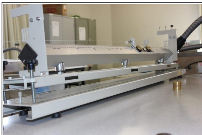
Figura 13.8 – O versátil trilho de ar é muito utilizado no LDF1. Muitos experimentos são efetuados neste equipamento, ligados à cinemática e mecânica.
